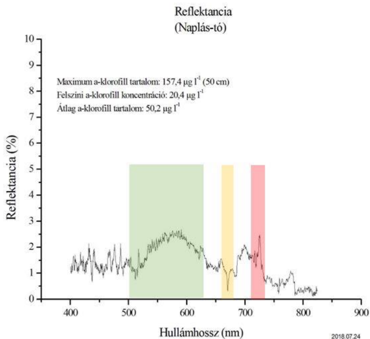
8. ábra Reflektancia görbe lefutása abban az esetben, ha az a-klorofill tartalom maximuma a 50 cm-nél mélyebben vízrétegben helyezkedett el
