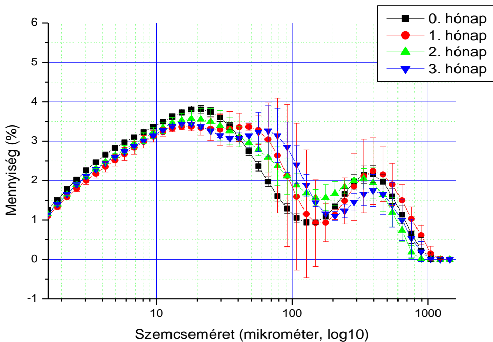
Melléklet, 31. ábra: A Magyarszombatfa-B minta szemcseméret-eloszlása, az adott szemcseméret tartomány százalékos értékével
