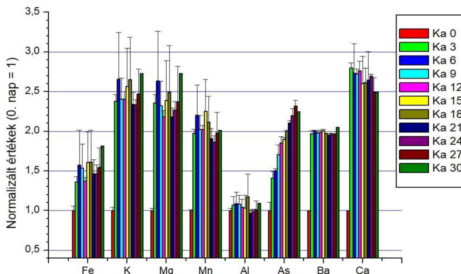
28. ábra: A talajextrakciós eredmények alakulása 30 napos érlelés (3 naponkénti mintavétel) esetében, a Keszthely-A mintán
