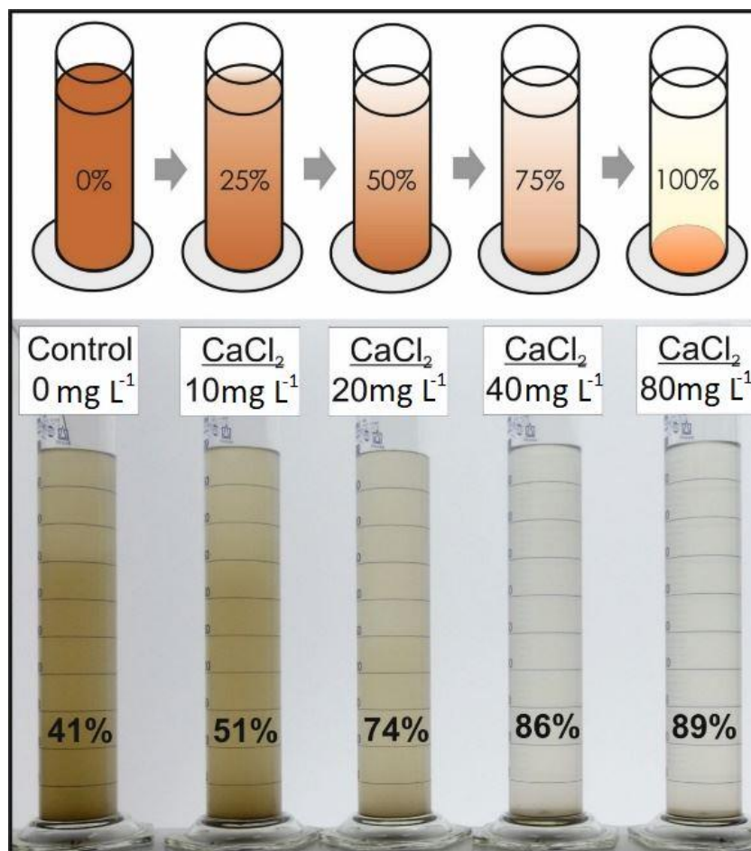
19. ábra: Az ülepedés hatékonysága, és a kísérleti elrendezés. Az oszlopokon feltüntetett százalékok a kiülepedés hatékonyságát jelzi, ahol a 0% a kezdeti szuszpenzió zavarossági értéke
