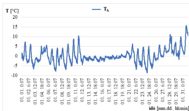
7. ábra, Hercegszántó HVB, külső hőmérséklet 2020 január hónapban
