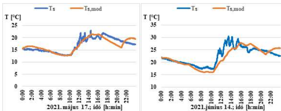
22. ábra, Modellezett T_{s,mod} és mért T_s belső hőmérsékletek validálás során
