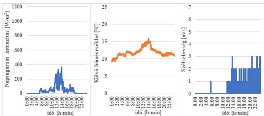
14. ábra, Napsugárzás, környezeti hőmérséklet és szélsebesség 2021. 05. 17.
