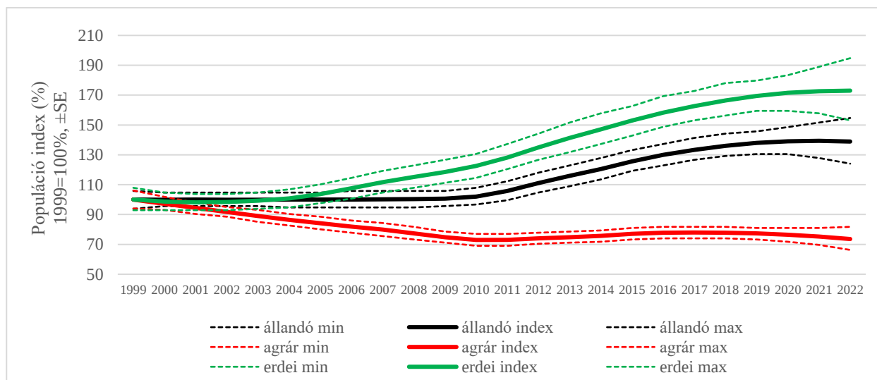
4. ábra Az egyes madárcsoportok szerinti biodiverzitásindikátor-értékek változása Magyarországon 1999 és 2022 között. A változás iránya és mértéke: „állandó” növekvő /Trend 1,9% ( \pm 0,2\% )/ ( p < 0,01 ) | „agrár” csökkenő /Trend 1,1% ( \pm 0,2\% )/ ( p < 0,01 ) | „erdei” növekvő /Trend 3,1% ( \pm 0,3\% )/ ( p < 0,01 ) (MME)
