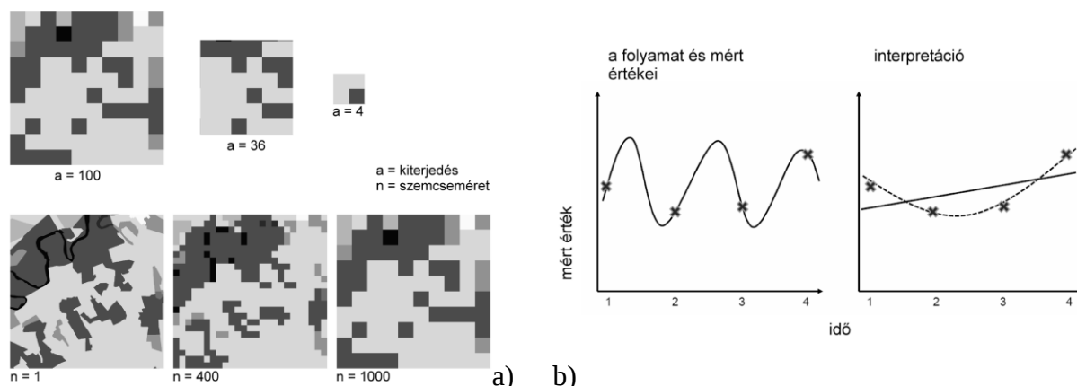
3. ábra A skálaprobléma két esete: a térbeli és az időbeli skála megválasztásának jelentősége (TURNER 1989 alapján MÁTÉ 2018)
