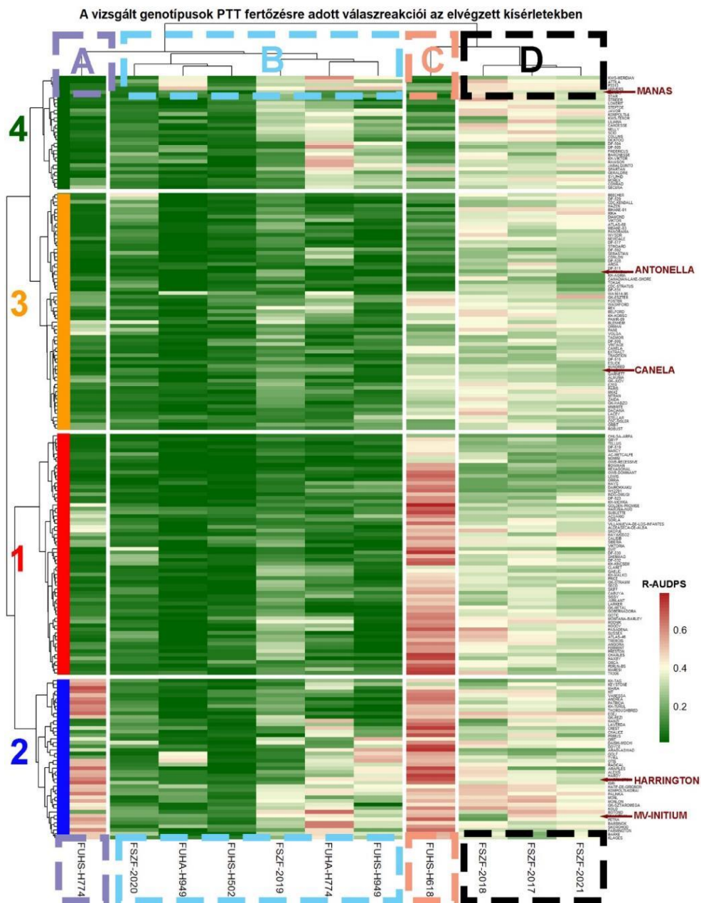
1. ábra: A 206 db árpa genotípus Pyrenophora sp. fertőzésre adott válaszreakciói (R-AUDPS) alapján készített elemzés az összes kísérletben. Az 5 vizsgált szabadföldi kísérleti év (2017, 2018, 2019, 2020, 2021), üvegházban felnőttkorban (H-774, H-949) és a fiatal korban (H-502, H-618, H-774, H-949) beállított kísérletek értékelése. Az A, B, C és D betűk a kísérletek klaszterekbe rendezését jelölik.
