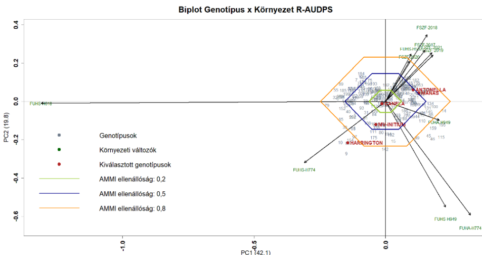
2. ábra: AMMI (Additive Main effects and Multiplicative Interaction) modell. A PC1 és PC2 tengelyek a genotípus x környezeti viszonyok összefüggését mutatják, zöld színnel a kísérletek, szürke színnel a 206 db vizsgált árpa genotípus és piros színnel az antioxidáns vizsgálatokra kiválasztott öt genotípus elhelyezkedése látható az origótól az R-AUDPS értékeik alapján.
