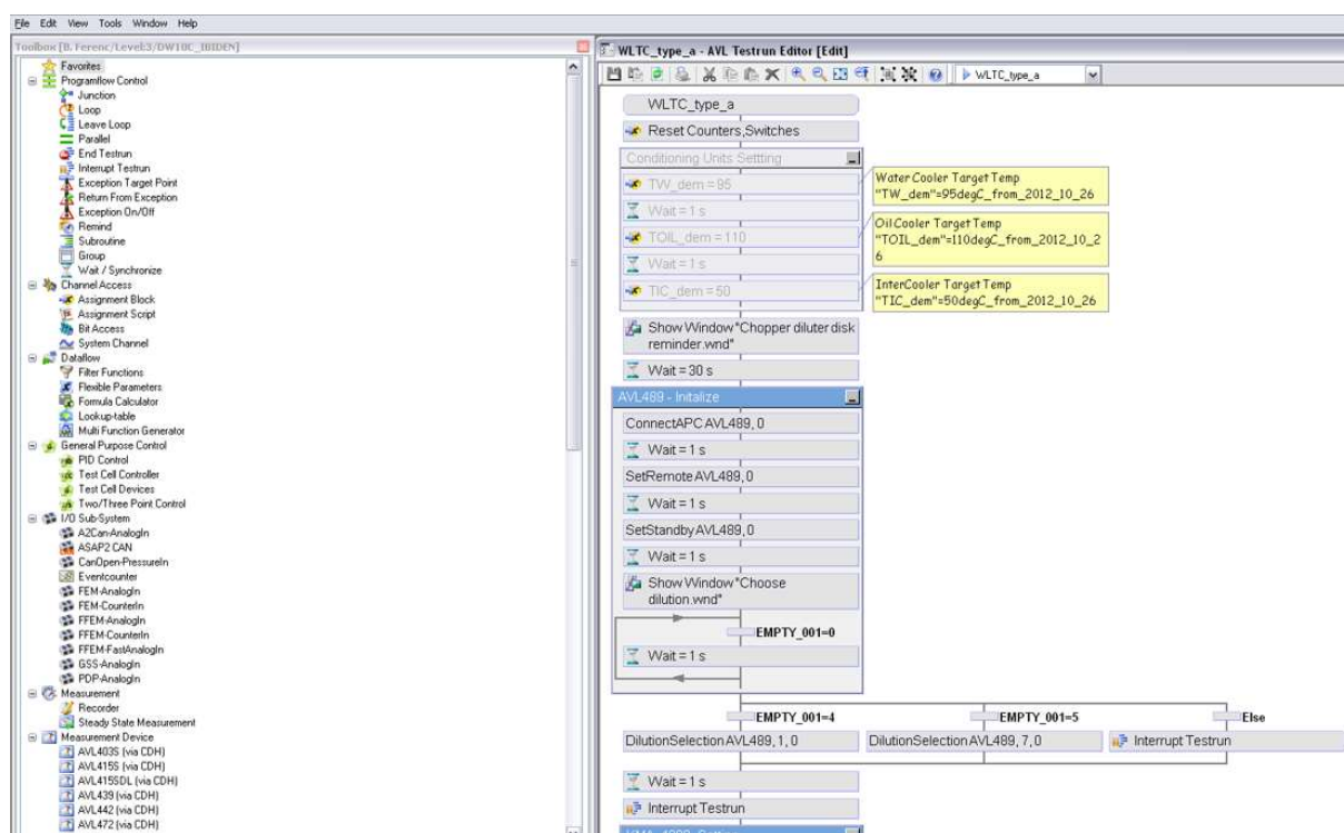
3.18. ábra AVL PUMA programozási felületen általam létrehozott WHSC parancssor (Forrás: Bíró Norbert)
