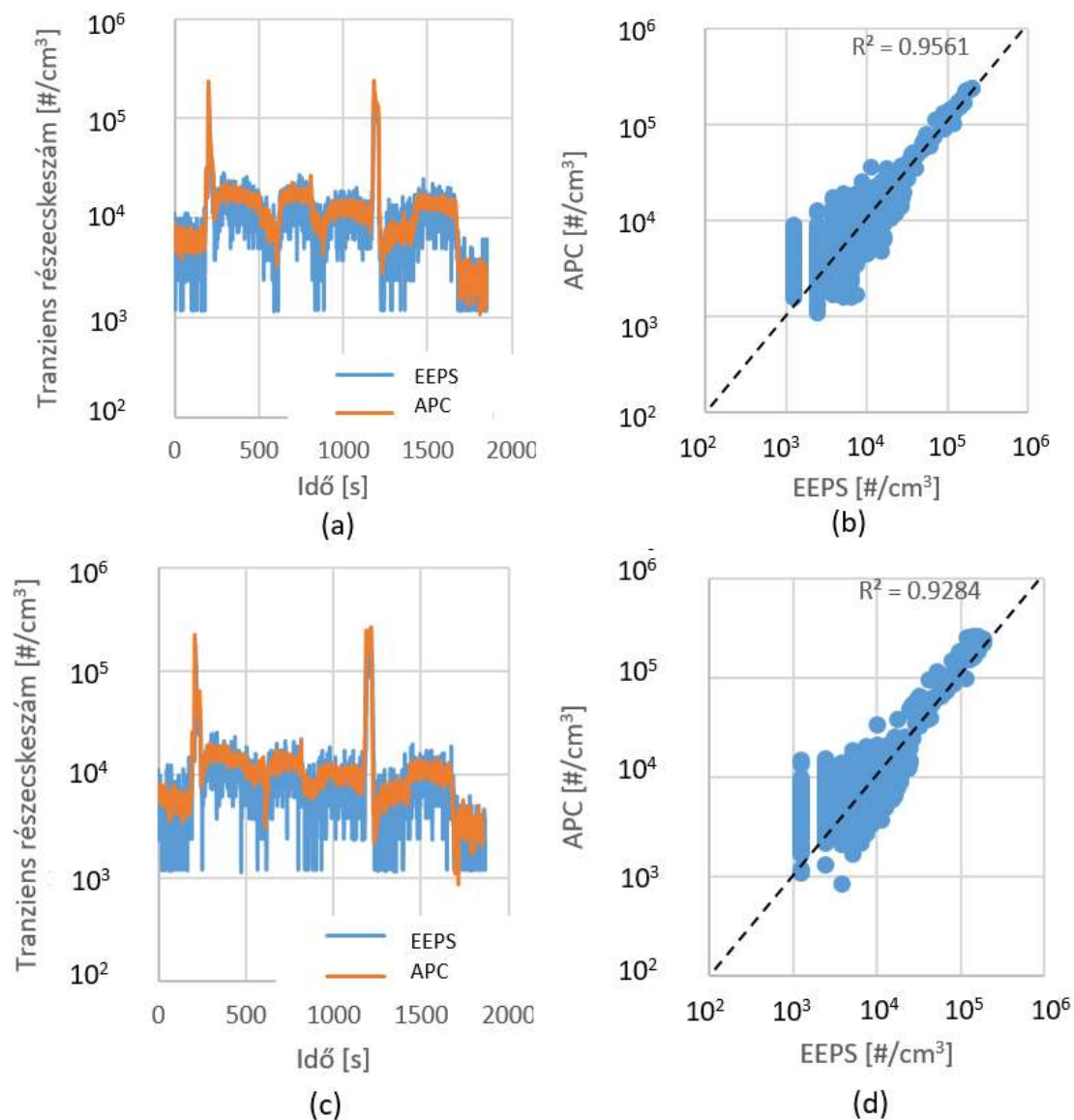
4.5. ábra Tranziens részecszekoncentráció (a), (c) és a részecske adatok lineáris regressziója (b), (d) kis részecszekoncentrációjú aeroszollal. (Forrás: Biró Norbert)
