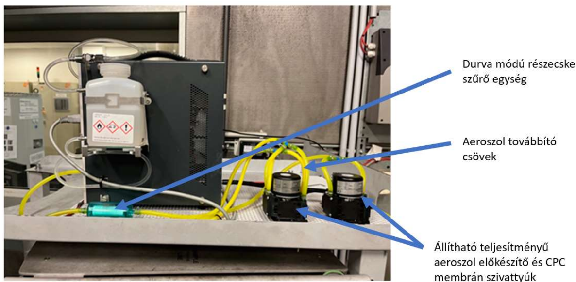
4.15. ábra A membránszivattyú és a durva módú részecske szűrő kivitelezése a CAD tervek alapján (Forrás: Bíró Norbert).
