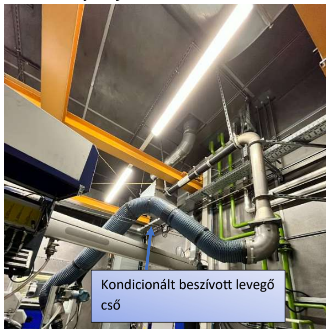
3.5. ábra Beszívott levegő csatlakozás a tesztmotorhoz (Forrás: Bíró Norbert)
