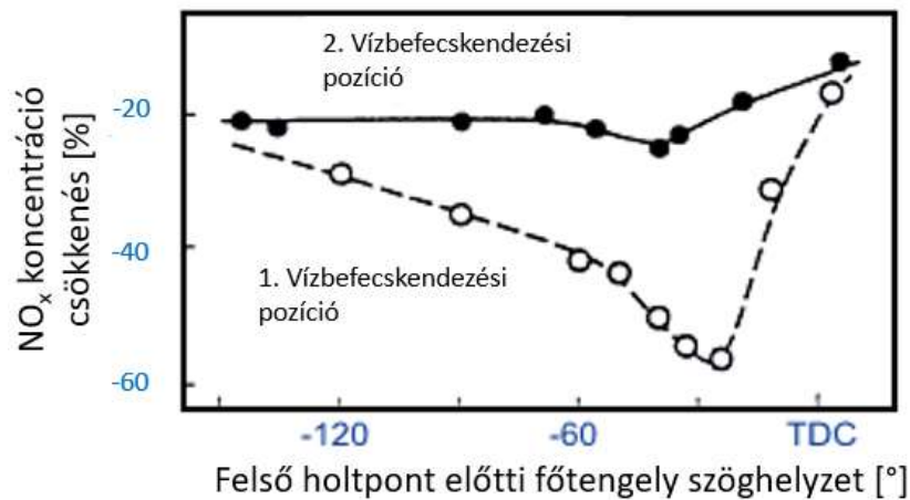
2.5. ábra A vízbefecskendezés hatása a \text{NO}_x emisszióra (Forrás: Miyamoto et al, 1995)
