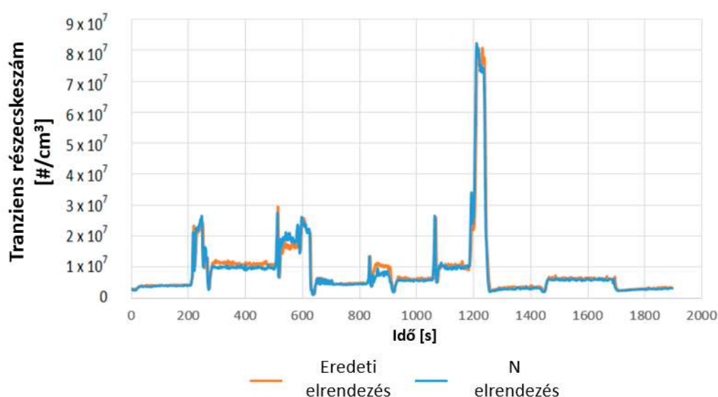
4.16. ábra Transziens részecskeszám WHSC ciklus alatt (Forrás: Bíró Norbert).
