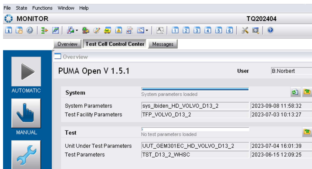
3.17. ábra Kísérleti paraméter kezelőfelület (Forrás: Biró Norbert)
