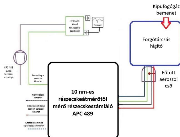
4.8. ábra Az APC 489 folyamatábrája eredeti elrendezéssel (Forrás: AVL GmbH).
