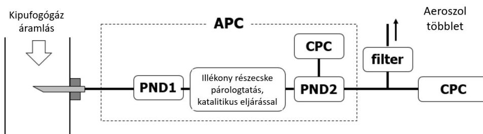
4.3. ábra 10 nm-es APC és 23 nm-es részecskéátmérőtől mérő CPC berendezésekből álló kísérleti kialakítás; APC = AVL részecskeszámláló; CPC = kondenzációs részecskeszámláló; PND = Részecskeszám-hígító. (Forrás: Bíró Norbert)
