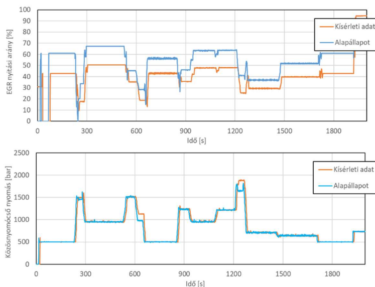
4.22. ábra Tranziens kipufogógáz visszavezetés aránya (EGR) és közösnyomócső nyomás a kísérleti WHSC ciklus alatt, összehasonlítva az alapállapottal (Forrás: Bíró Norbert).
