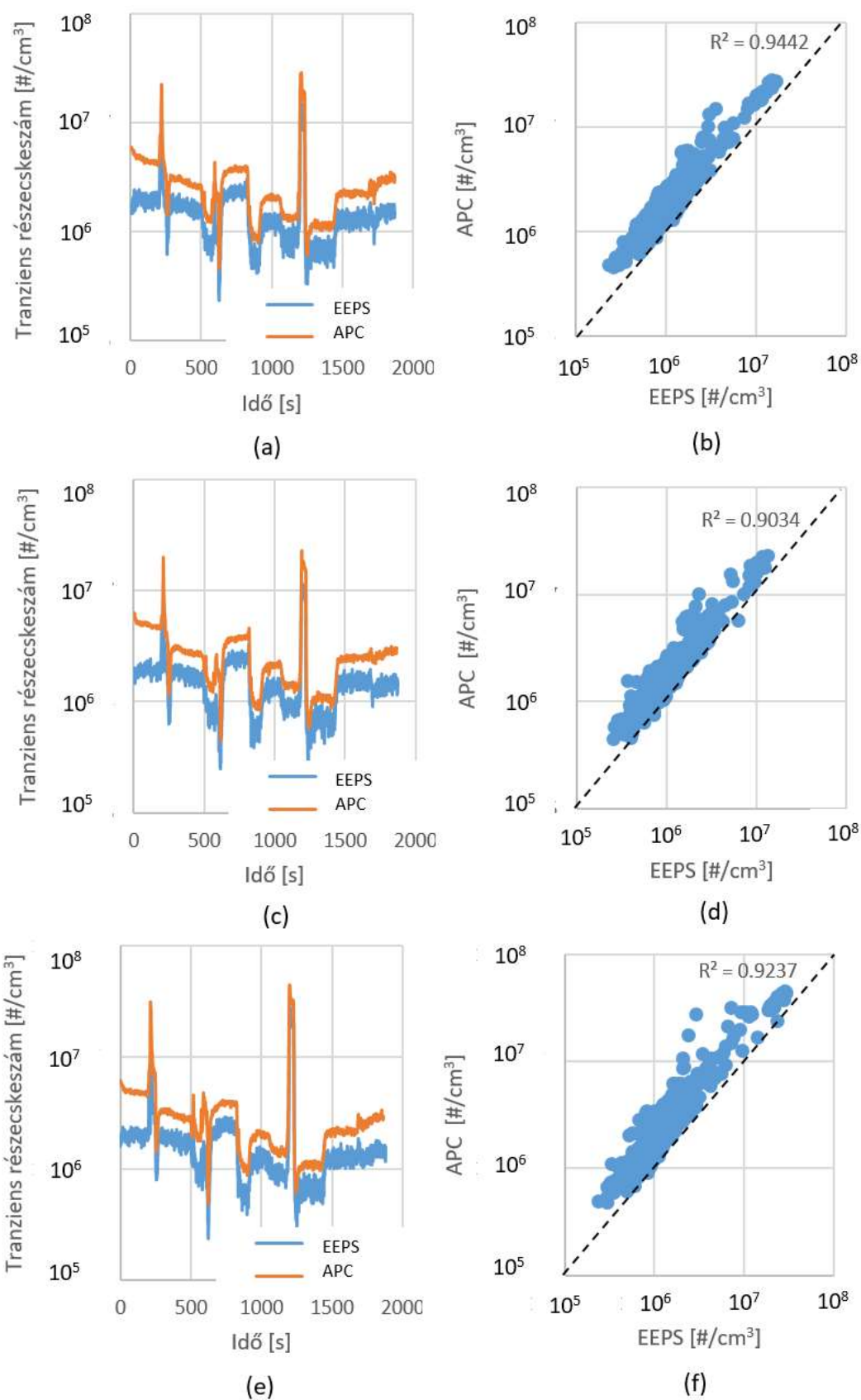
4.4. ábra Tranziens részecskekoncentráció (a), (c), (e) és a részecske adatok lineáris regressziója (b), (d), (f) nagy részecskekoncentrációjú aeroszollal. (Forrás: Bíró Norbert)
