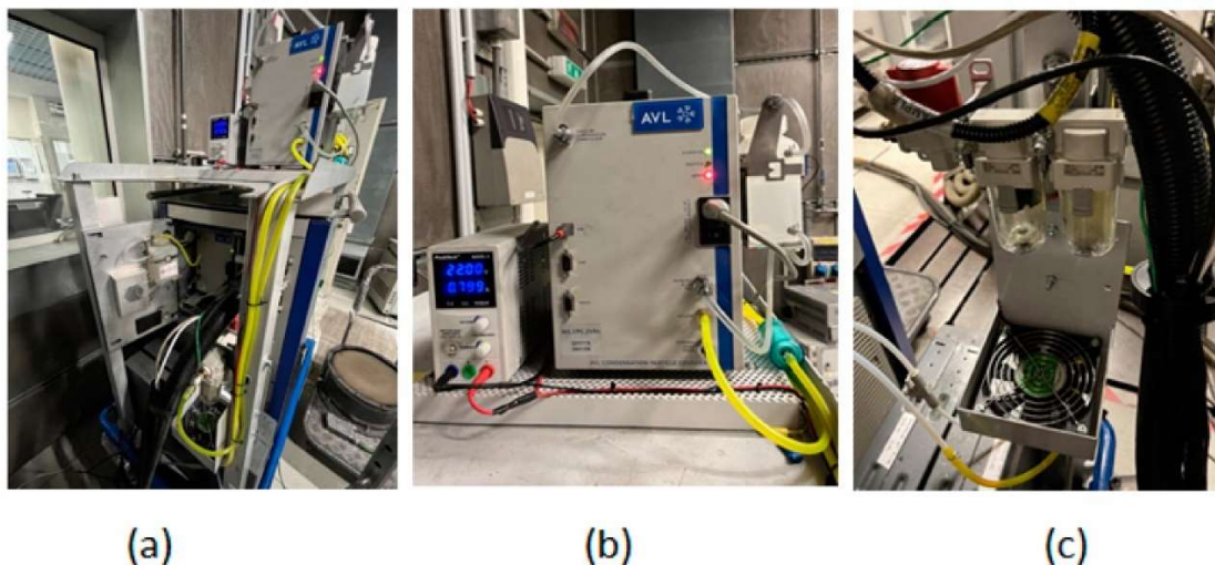
4.14. ábra APC 489 N-elrendezéssel (a), CPC 488 és az állítható tápegység (b), valamint kondenzátum egységgel és hűtőventilátorral (c) kivitelezése a CAD tervek alapján (Forrás: Bíró Norbert).
