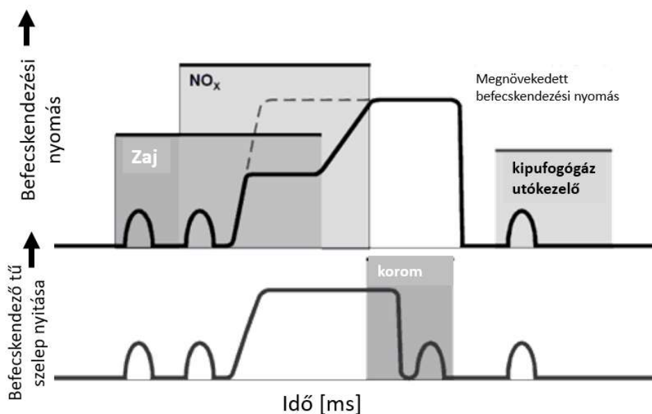
2.8.ábra Többszörös befecskendezés hatása a káros emissziókra
