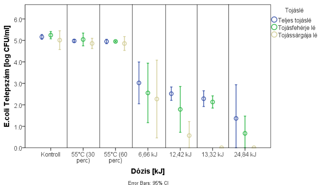
30. ábra: Telepképző baktériumszám logaritmus értékének (log CFU/ml) változása az kombinált ultrahangos kezelési dózis függvényében
