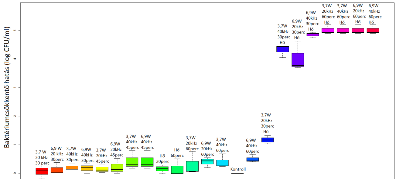
44. ábra: A kezelések baktericid hatásának boxplot eredményei tojássárgája lében
