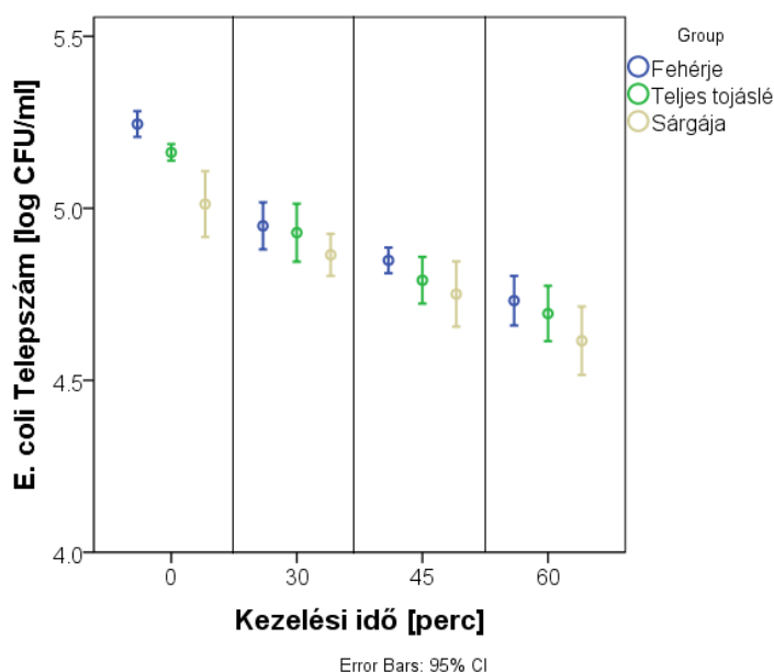
13. ábra: Telepképző baktériumszám logaritmus értéke (log CFU/ml) változása az ultrahangos kezelés kezelési idejének függvényében
