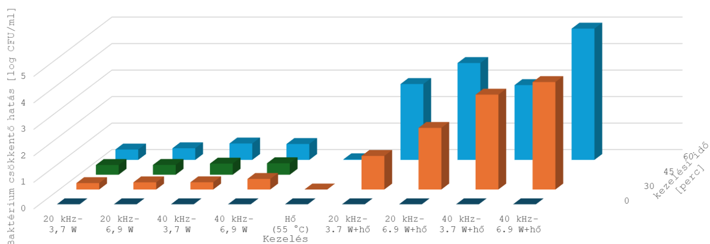
37. ábra: A különböző kezelések baktericid hatása tojásfehérje lé esetében
