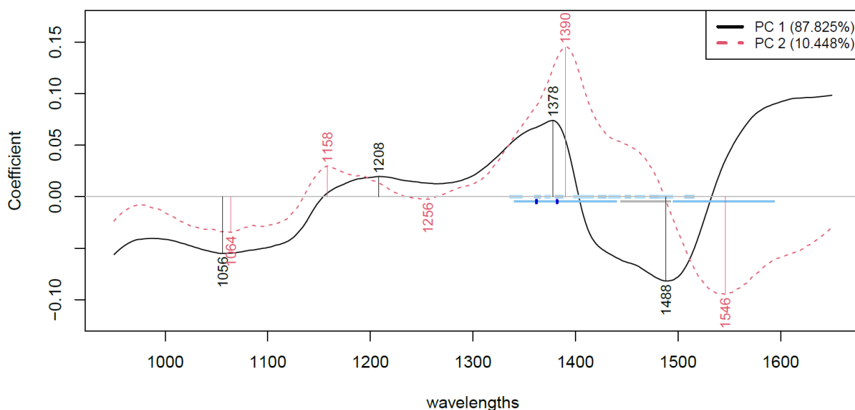
16. ábra: A PC1 és PC2 főkomponens kialakulásához hozzájáruló hullámhosszok, tojástermekként (a. – tojásfehérje lé, b. – tojássárgája lé, c. – teljes tojáslé)
