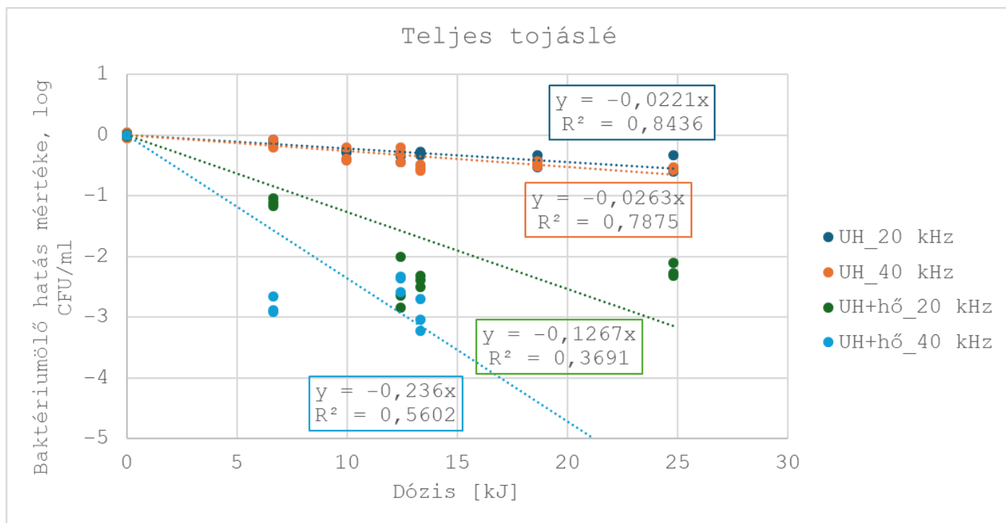
42. ábra: Baktériumölő hatás és dózis kapcsolatának modelljei az önálló ultrahangos kezelés és a kombinált kezelés esetében 20 kHz és 40 kHz vonatkozásában teljes tojásle esetében
