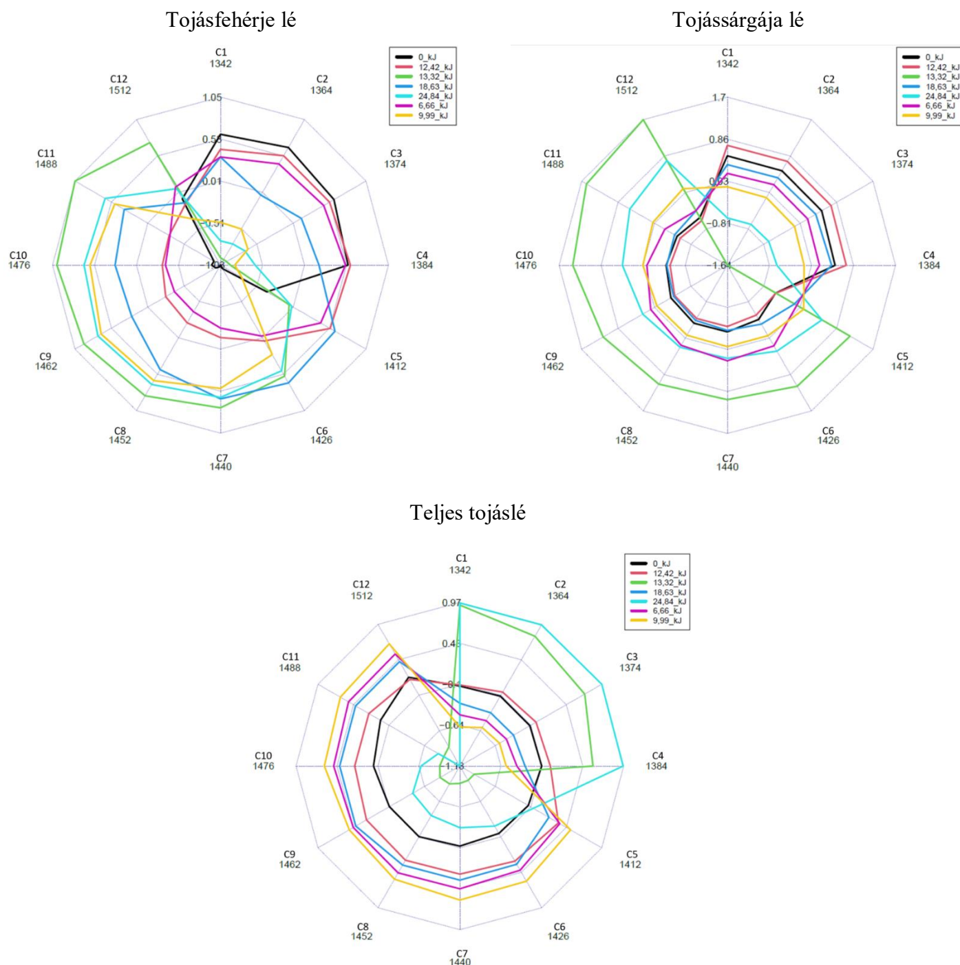
26. ábra: A kezelés dózisának Aquagramjai - WASP ( Tojásfehérje lé; Tojássárgája lé; Teljes tojáslé)
