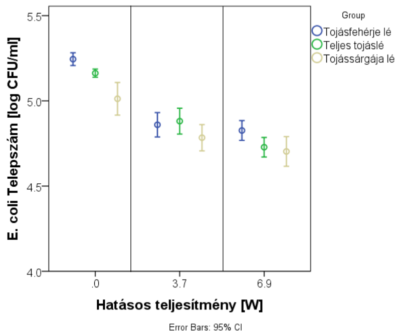
11. ábra: Telepképző baktériumszám logaritmus értékek (log CFU/ml) változása az ultrahangos kezelés hatásos teljesítményének függvényében
