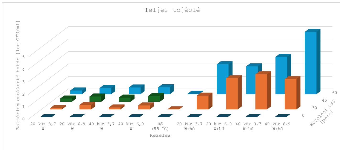
39. ábra: A különböző kezelések baktericid hatása teljes tojászlé esetében
