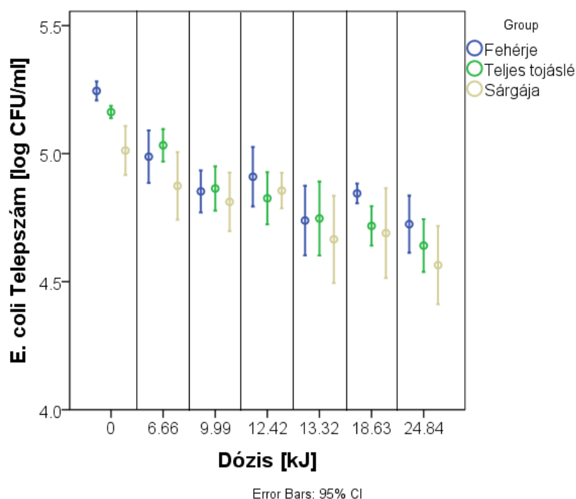
14. ábra: Telepképző baktériumszám logaritmusos értékének (log CFU/ml) változása az ultrahangos kezelés dózisének függvényében
