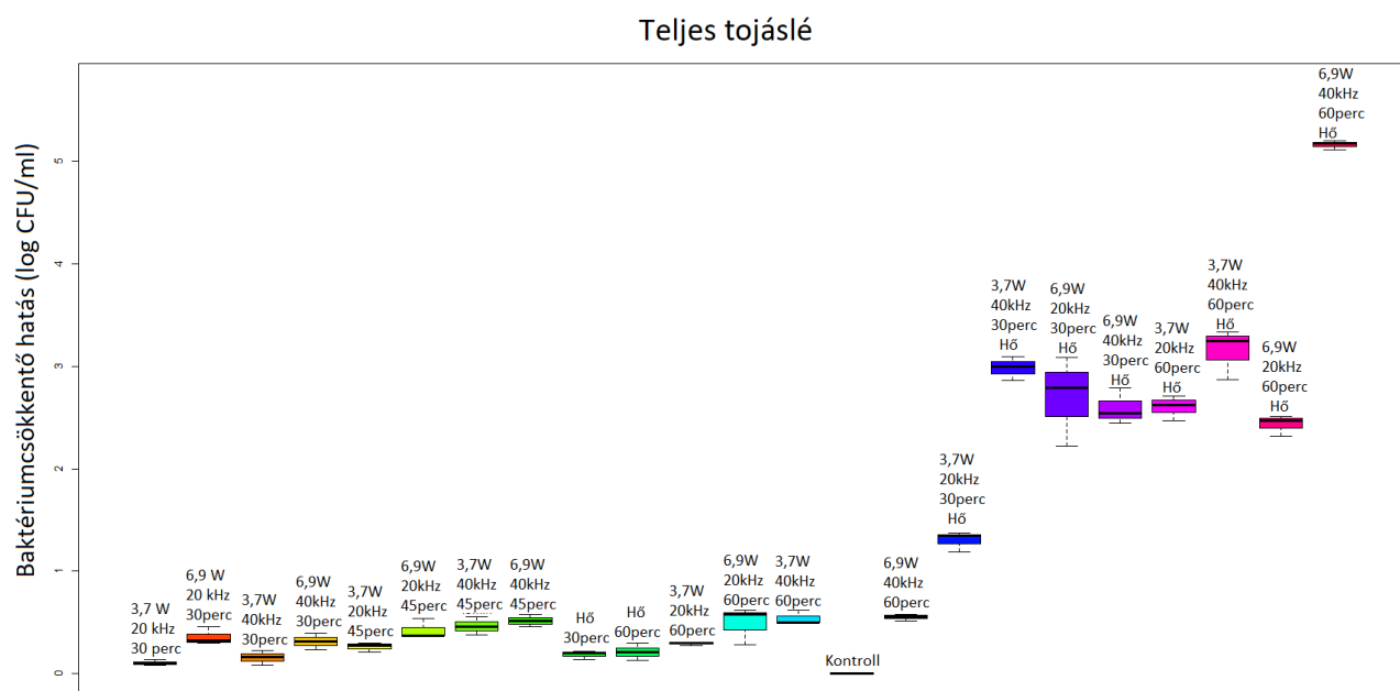
45. ábra: A kezelések baktericid hatásának boxplot eredményei teljes tojászlében
