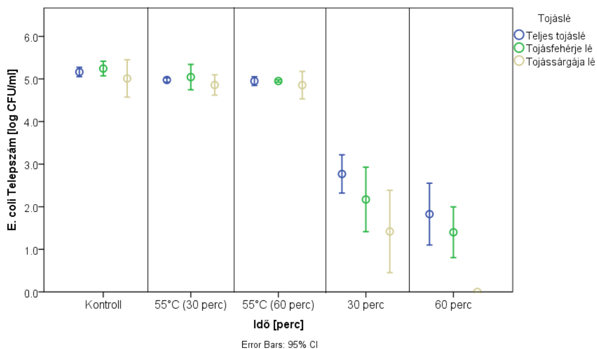
29. ábra: Telepképző baktériumszám logaritmikus értékének (log CFU/ml) változása az kombinált ultrahangos kezelési idő függvényében
