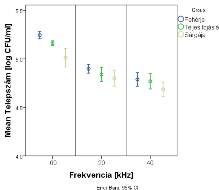
12. ábra: :: Telepképző baktériumszám logaritmus értéke (log CFU/ml) változása az ultrahangos kezelés frekvenciájának függvényében
