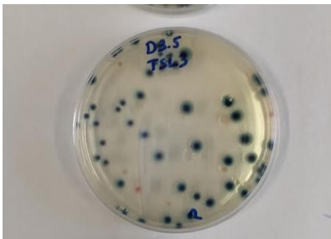
9. ábra: Szelektív agar, E. coli jelenlétét kék színnel jelzi
