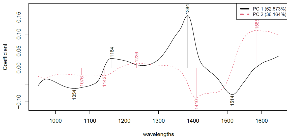
46. ábra: Főkomponensek kialakulásához hozzájáruló hullámhosszok koefficiensei (a – tojásfehérje lé; b – tojássárgája lé; c – teljes tojáslé)
