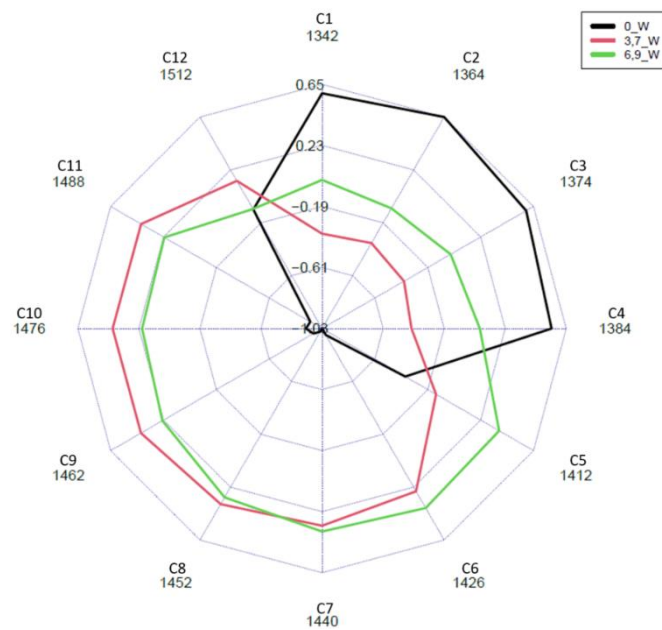
23. ábra: A kezelés hatásos teljesítményének Aquagramja – WASP (tojásfehérje lé)
