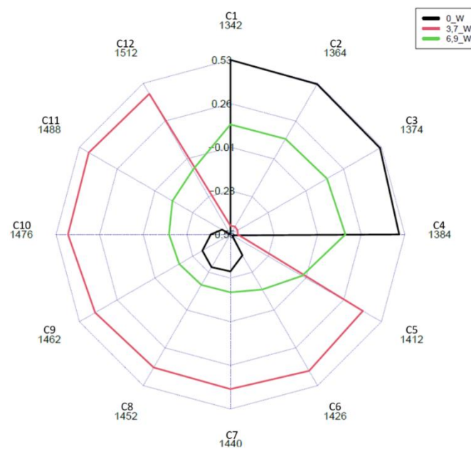
24. ábra: A kezelés hatásos teljesítményének Aquagramja – WASP (tojássárgája lé)
