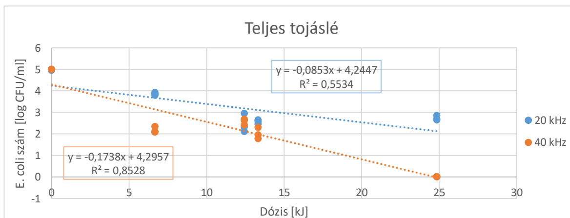
31. ábra: A koncentráció (y) regressziója a kezelés energiadóziséval (x) 20 kHz és 40 kHz esetén (a. - tojásfehérje, b. - tojássárgája, c. - teljes tojásle).
