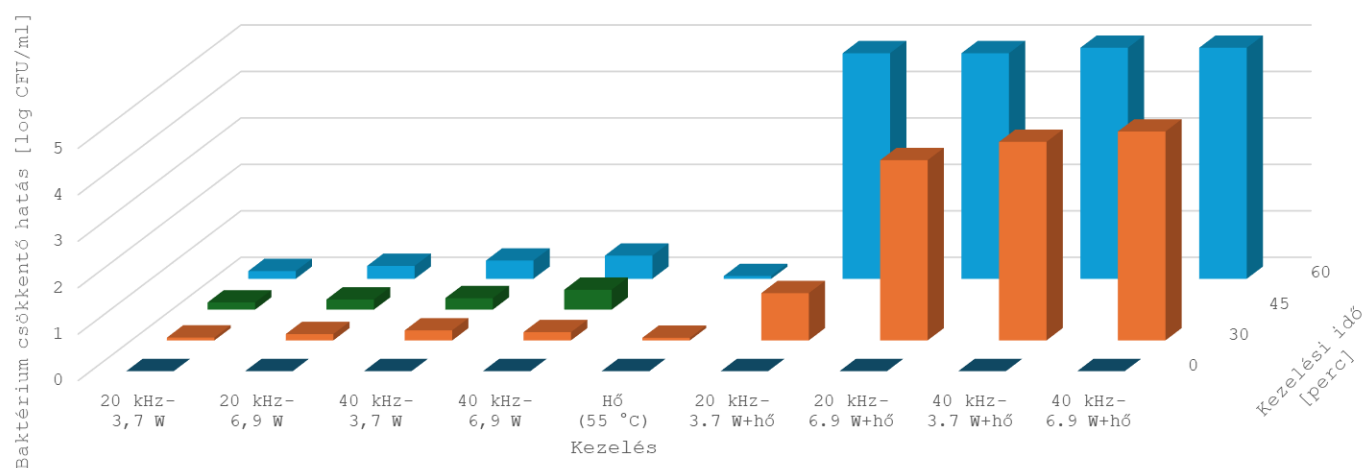
38. ábra: A különböző kezelések baktericid hatása tojássárgája lé esetében
