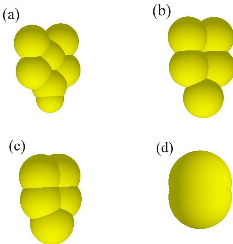
2.4. ábra: A diszkrét elemes szimulációkban szereplő szemcsealakok: (a) lapos, (b) hosszúkas, (c) szögletes, (d) kerek
