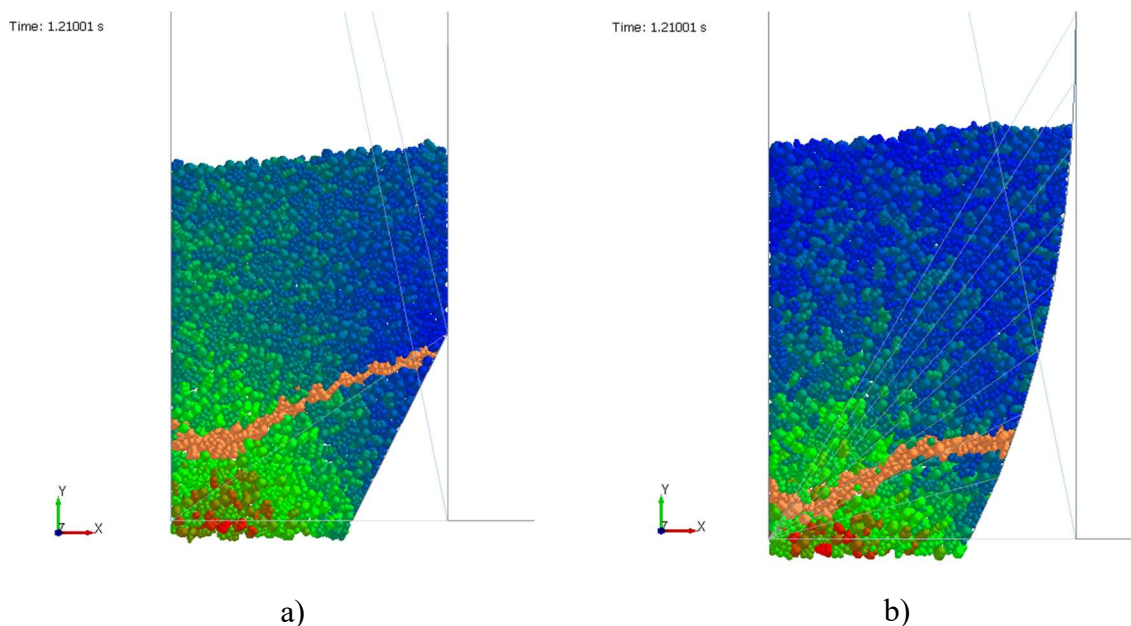
2.10. ábra: A középén elhelyezett festett sávok alakja a) egyenes, illetve b) ciklois alakú lamella esetén \Delta t = 0,21 s elteltével
