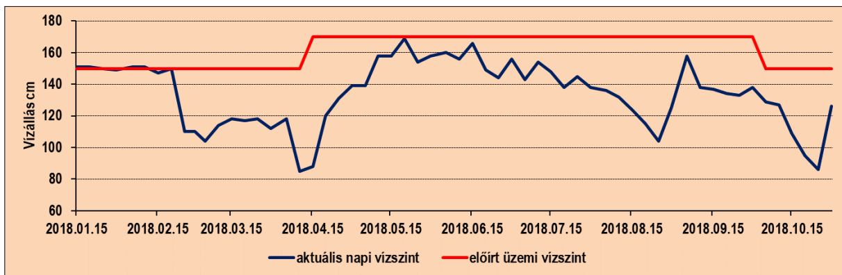
6. ábra: Az RSD Kvassay-zsilipnél lévő 121028 számú felszíni vízrajzi állomás vízállás adata az előírt üzemi vízszinthez képest a 2018. évben (forrás: OVF)
