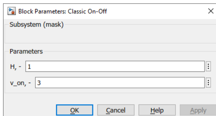
4.32. ábra A kétállású szabályozó alrendszer beállítható paraméterei
