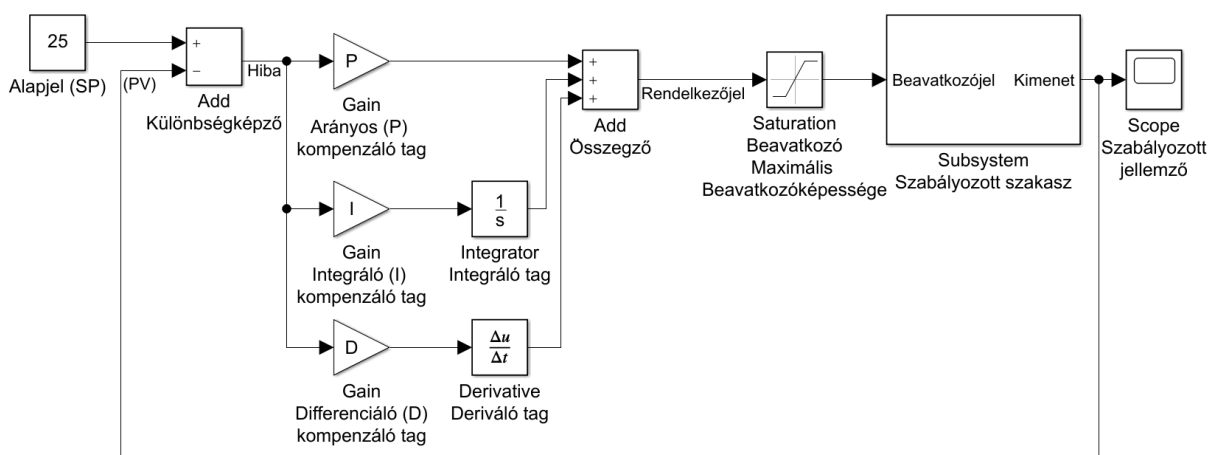
3.11. ábra A PID szabályozóval kialakított szabályozási kör felépítése MATLAB-Simulink környezetben
