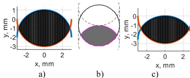
4.13. ábra Áramlási keresztmetszet \varphi = 30^\circ -nál, a) SS-modell: 16,50 \text{ mm}^2 , b) CAD: 11,37 \text{ mm}^2 , c) ET-modell: 11,37 \text{ mm}^2
