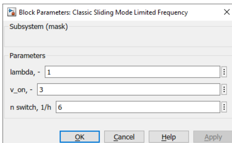
4.49. ábra A limitált beavatkozási frekvenciájú csúszómód-szabályozó alrendszer maszkon beállítható paraméterei
