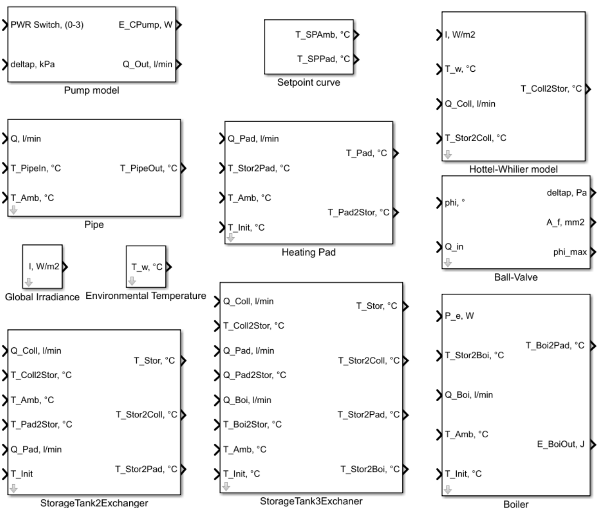
4.64. ábra A kiegészített keretrendszer modellkönyvtára
