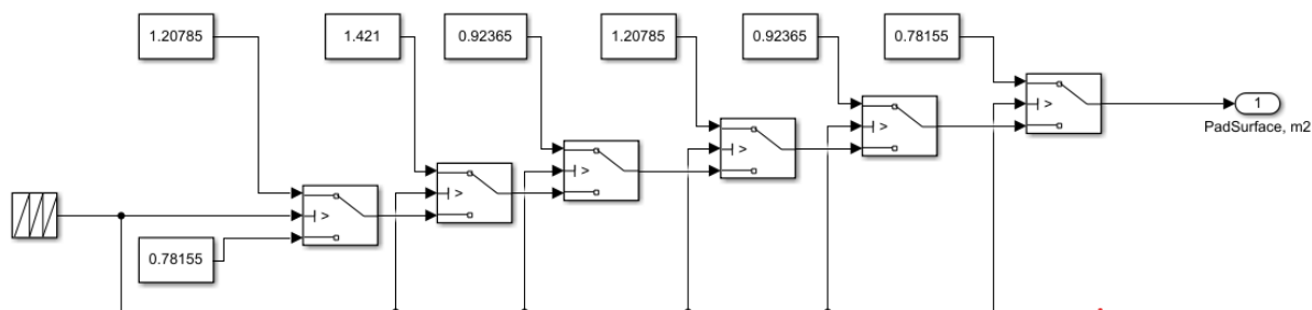
4.100. ábra A fűtőlapok szabad felületét meghatározó modell
