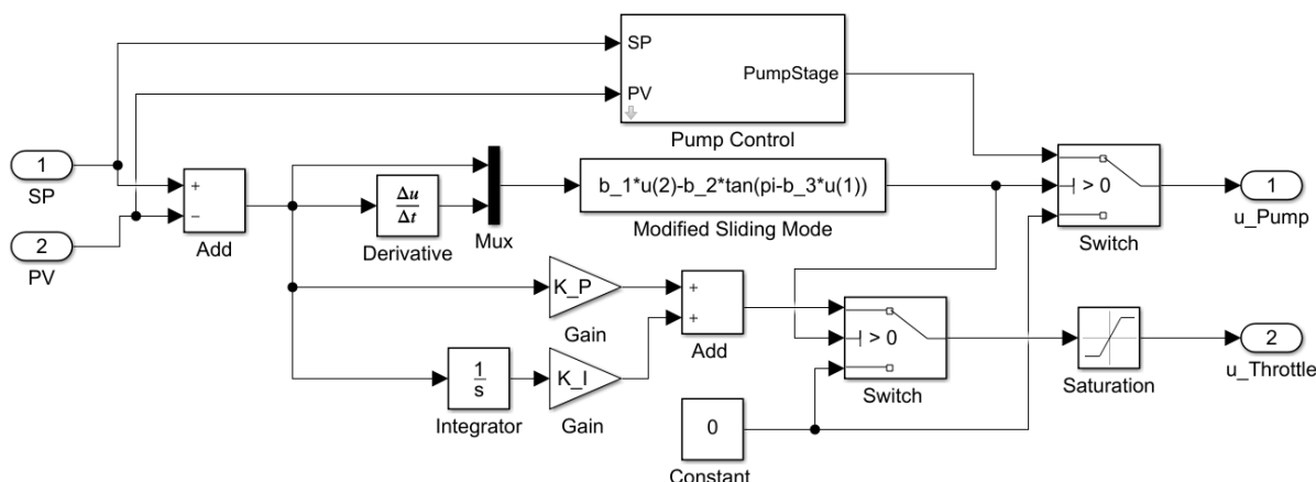
4.63. ábra A kombinált módosított csúszómód-szabályozó felépítése
