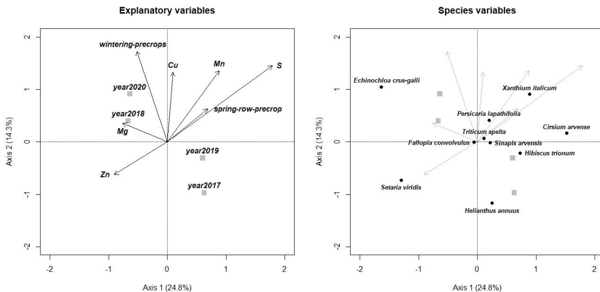
3. ábra. A redundancia analízis (RDA) modell ordinációs diagramjai fénymag kultúrában (Nyíl: numerikus változó; négyzet: faktoriális évváltozó; kör: faj).
