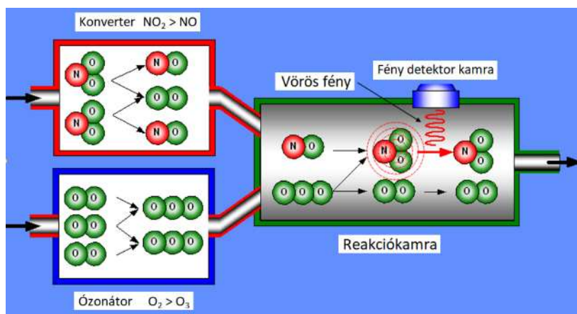
3.8. ábra: A Kemilumineszcens detektor sematikus ábrája
