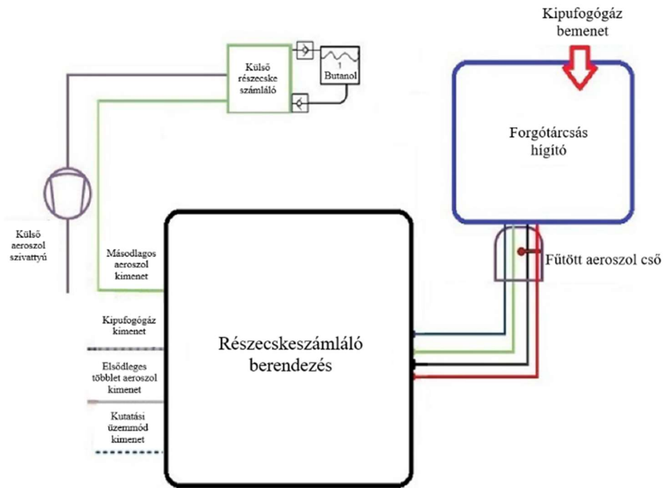
3.2. ábra: APC 489 vázlatos rajza
