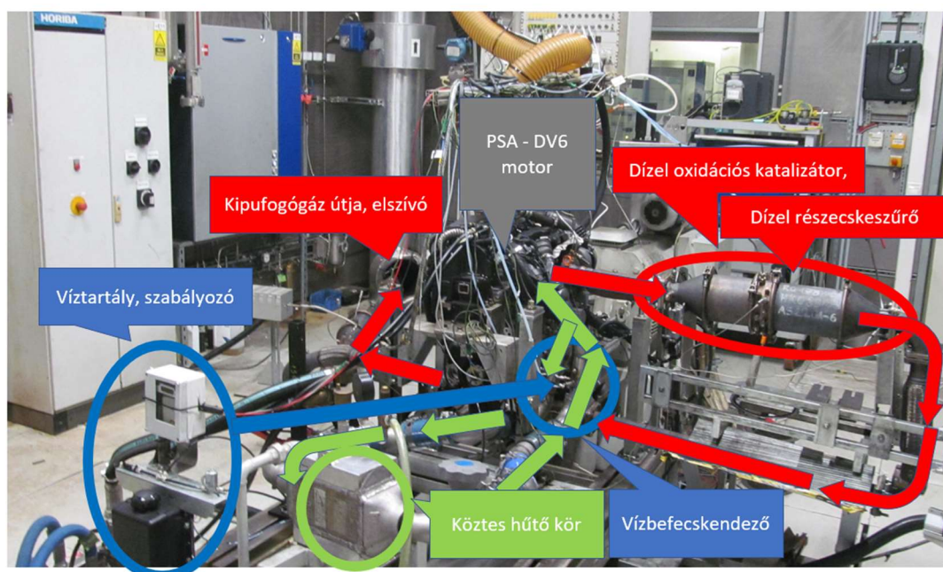
3.16. ábra: Tesztcella a teljes mérőrendszerrel
