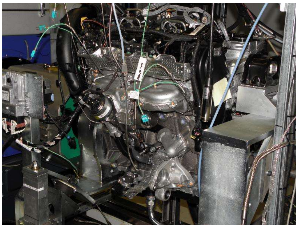
3.18. ábra: PSA DW10 motor, AVL PC Load System 220kW motorfékpadra telepítve.
