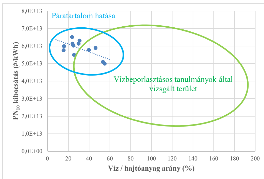
4.14. ábra: A részecskeszám eredmények a víz/hajtóanyag arány függvényében, a vízbefecskendezéses vizsgálatok jellemző tartományával
