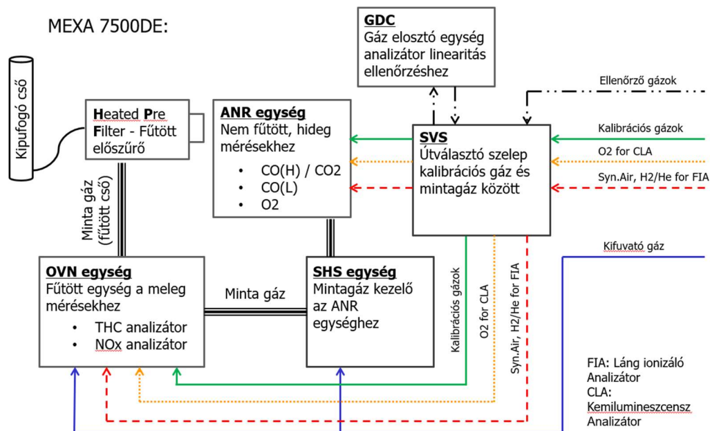
3.7. ábra: HORIBA MEXA 7500 kipufogógáz analizáló berendezés teljes sematikus gázáram ábrája
