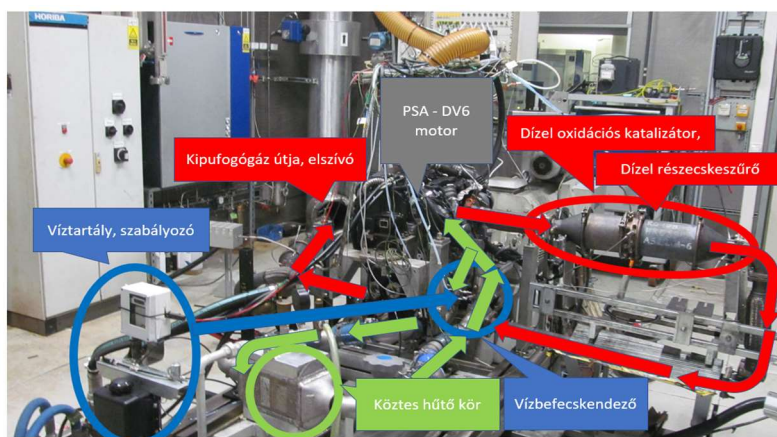
2.3. ábra: Tesztcella a teljes mérőrendszerrel
